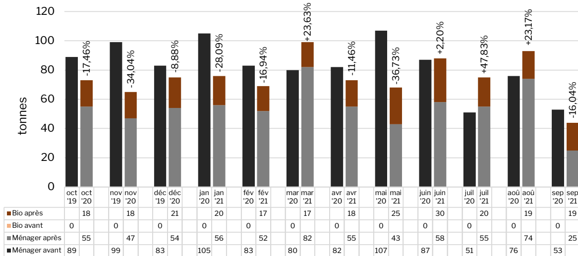
Graphique 12 : Variation des quantités collectées par poubelle déchets ménagers résiduels et biodéchets
