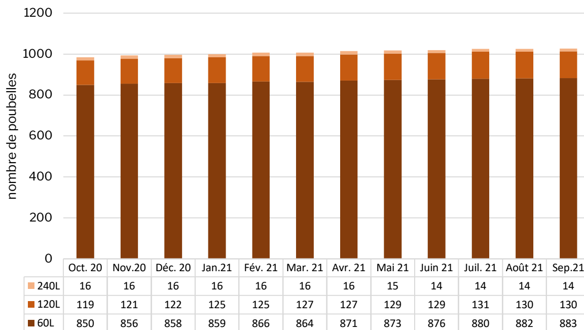
Graphique 3 : Evolution du nombre de poubelles biodéchets en circulation
