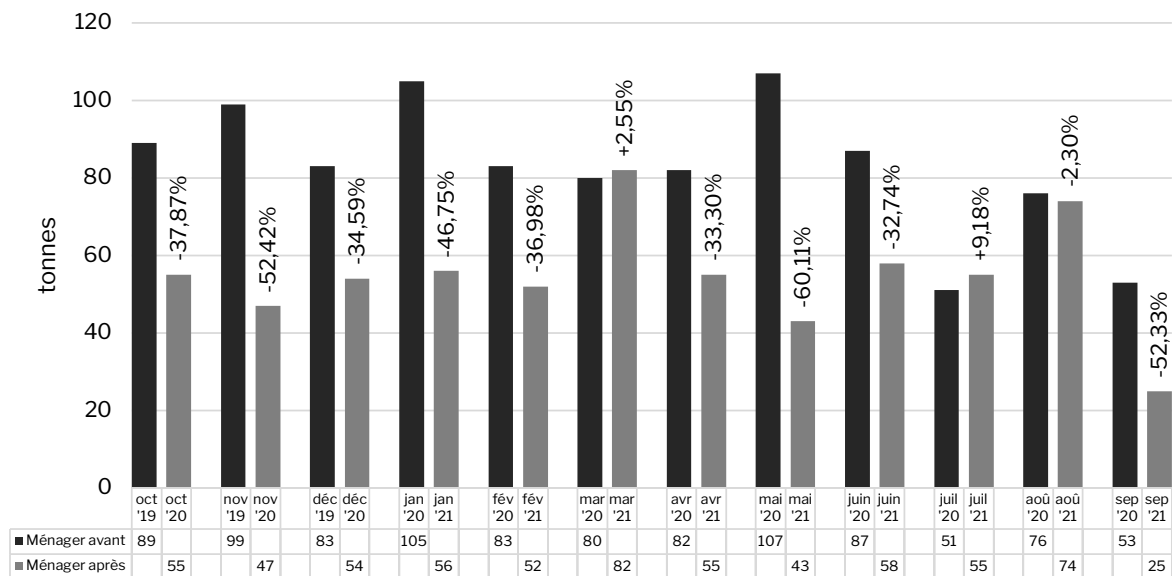
Graphique 11 : Variation des quantités collectées par poubelles pour déchets ménagers résiduels
