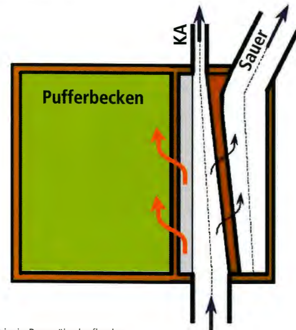
Prinzip Regenüberlaufbecken
