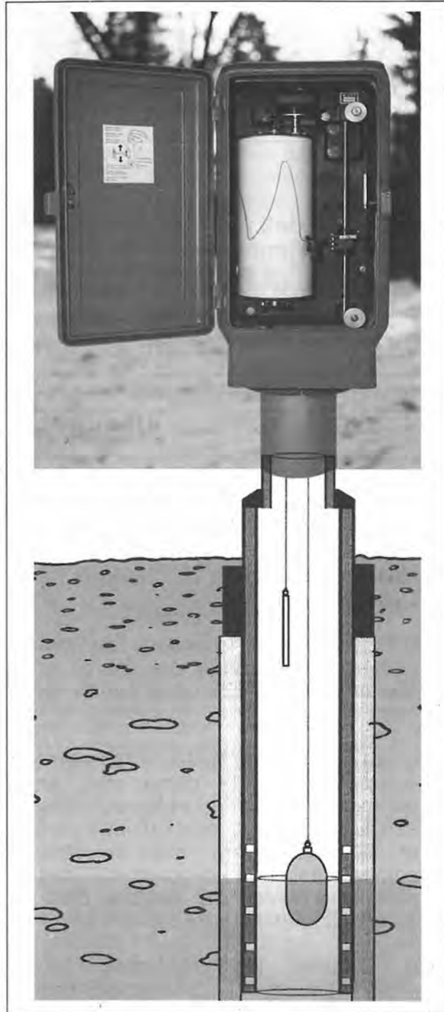
Station limnimétrique (coupe)
